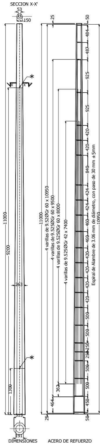
FIGURA 4- Poste PCRGR60-11-700
